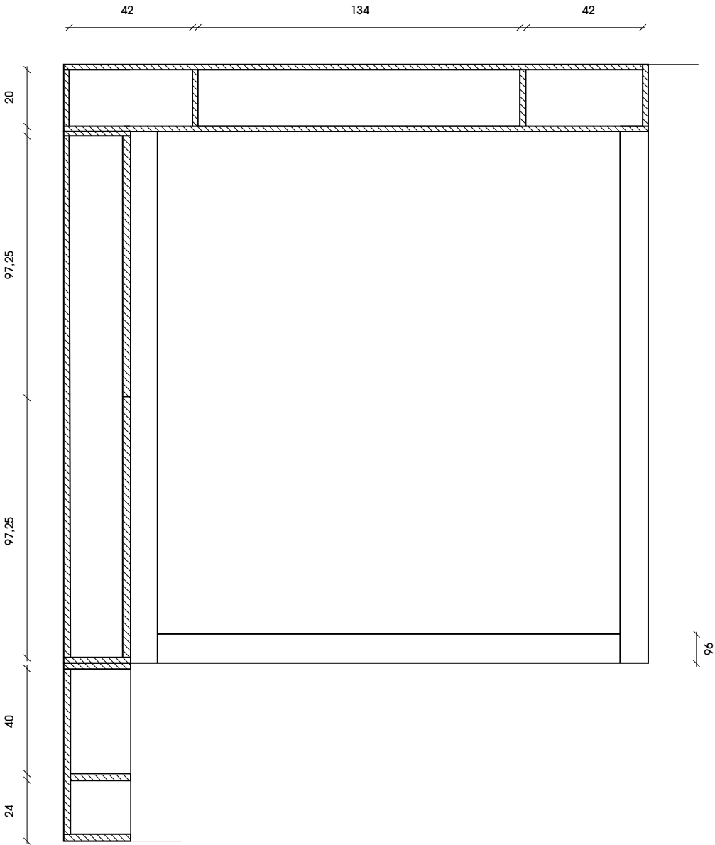
CORTE CD
