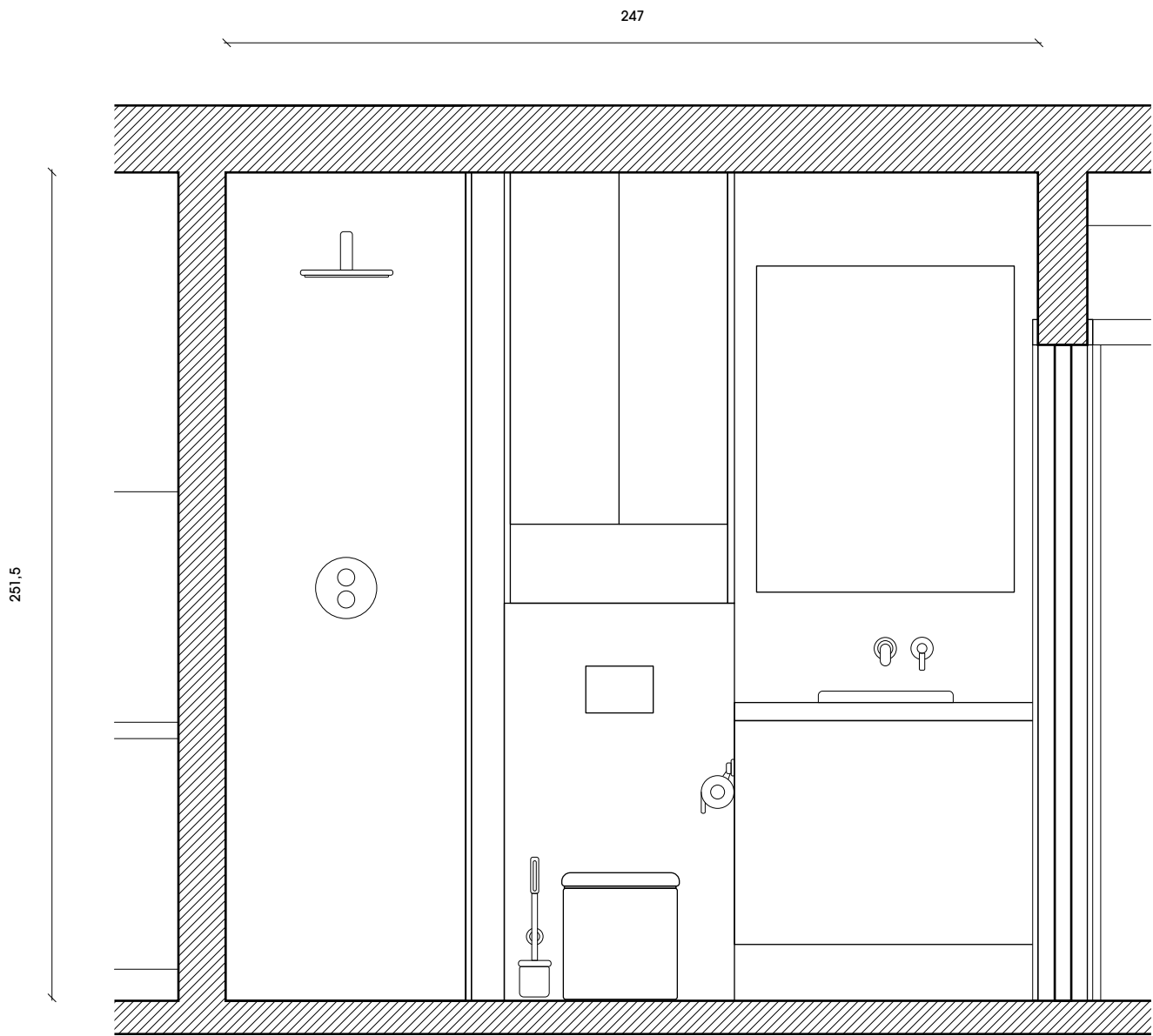
CORTE AB
