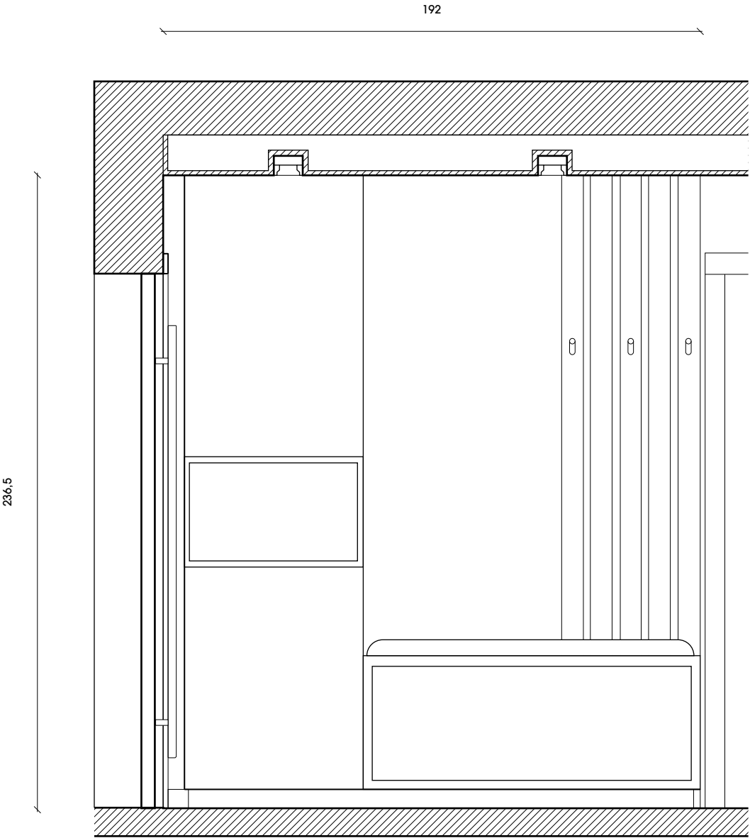
CORTE AB
