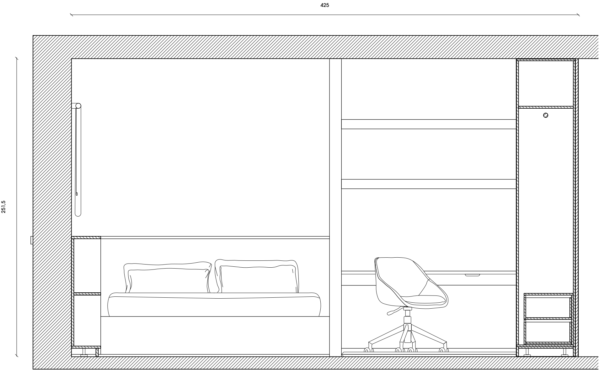
CORTE AB
