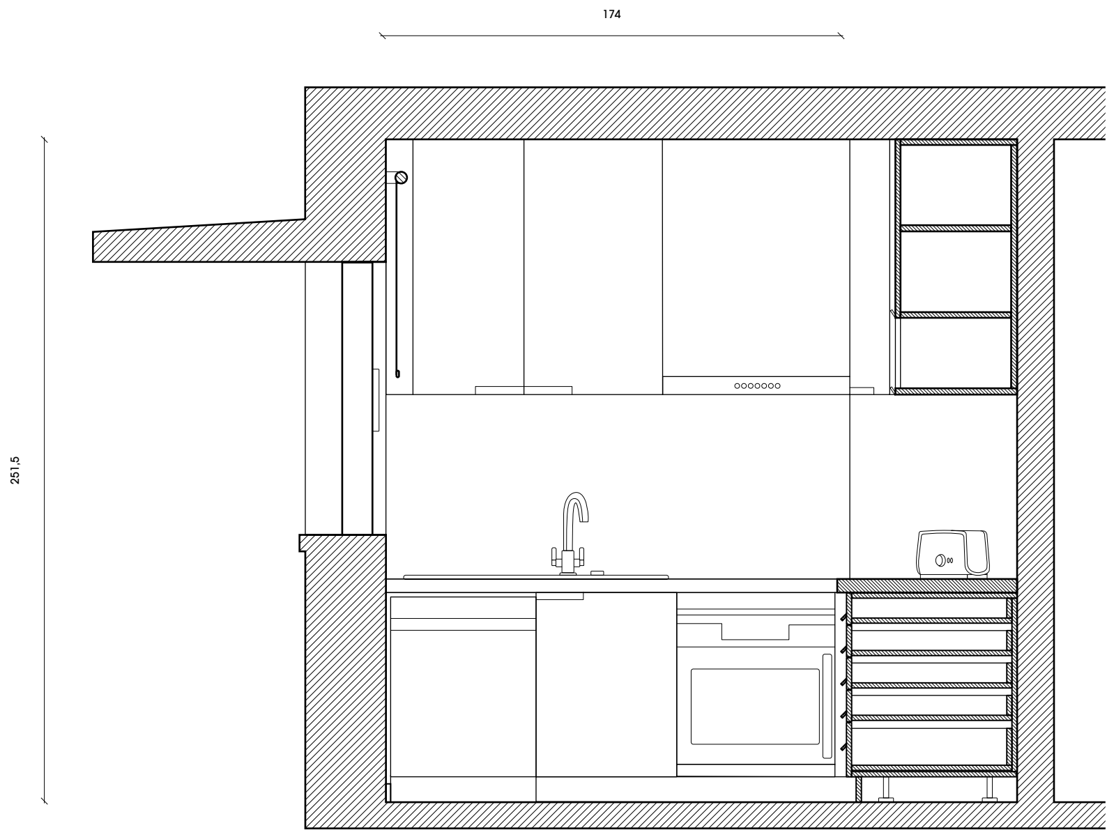
CORTE AB
