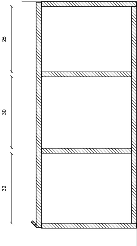
CORTE AB
