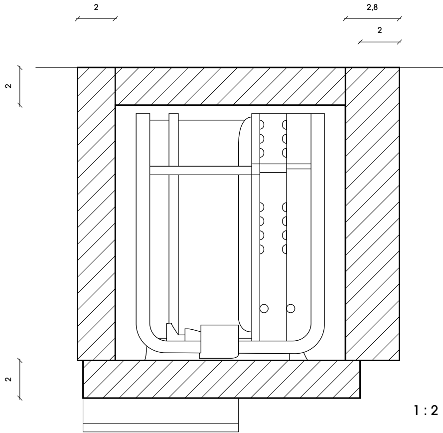
CORTE CD
