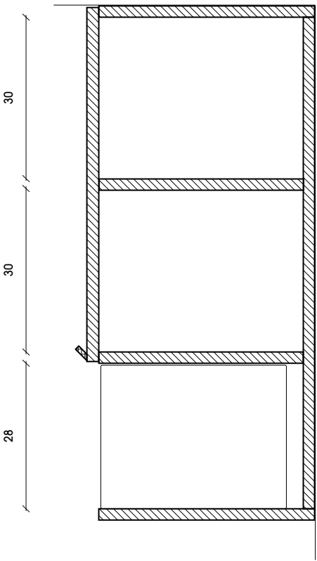
CORTE AB
