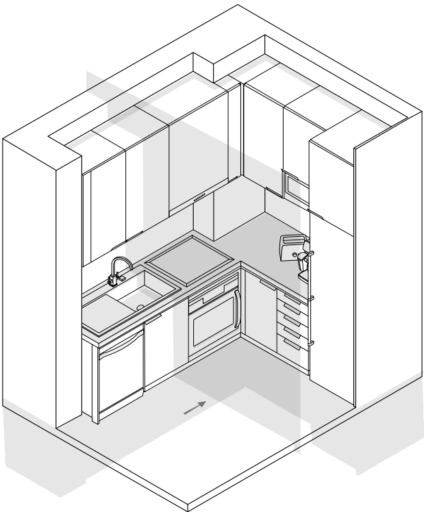
Medidas em cm
