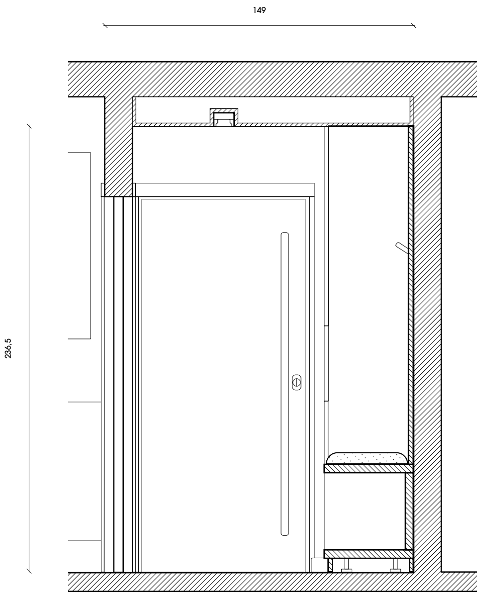
CORTE CD
