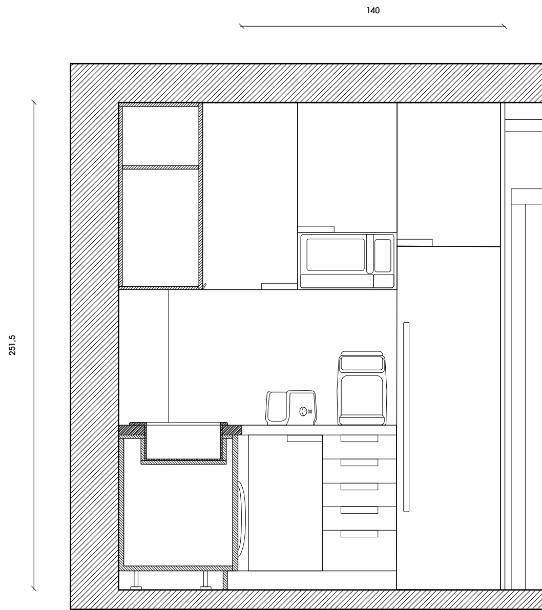
CORTE CD
