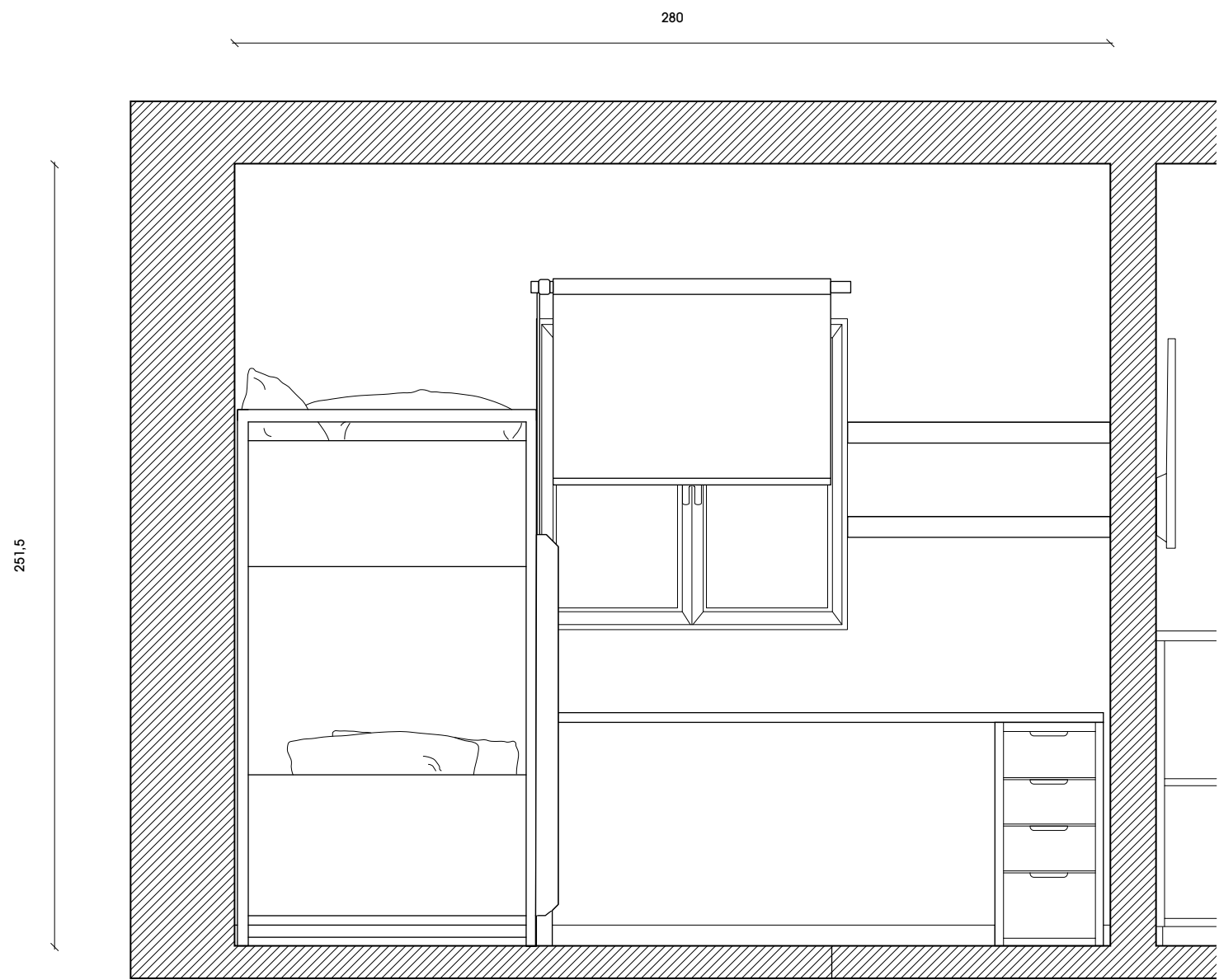
CORTE CD
