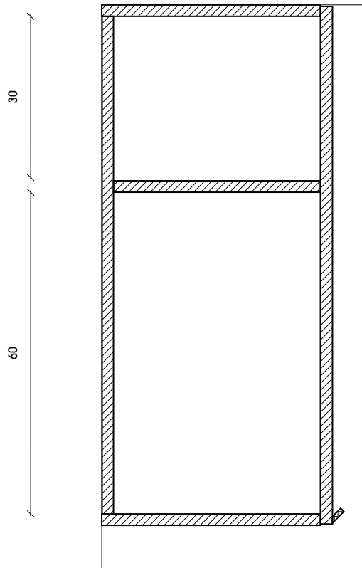
CORTE AB
