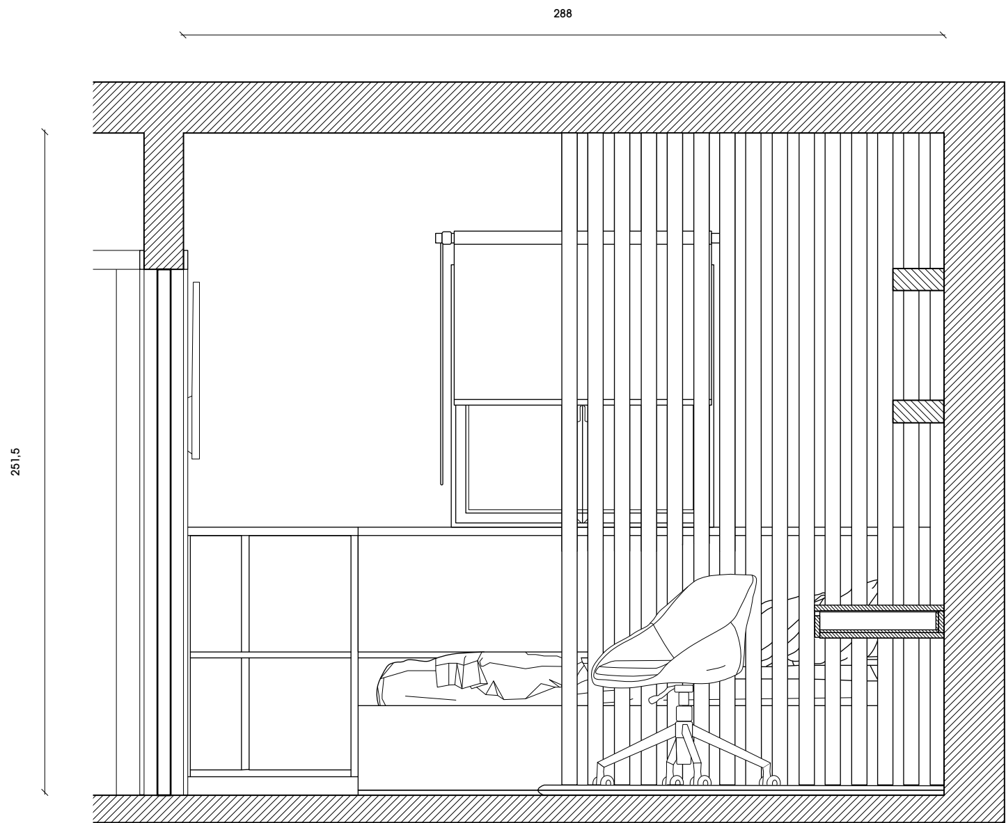
CORTE CD
