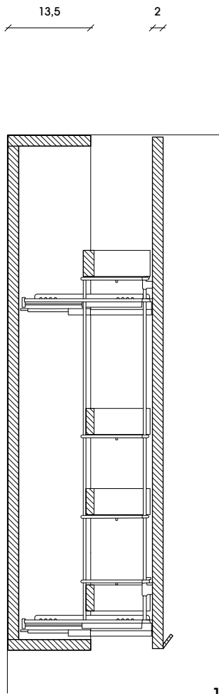
CORTE AB
