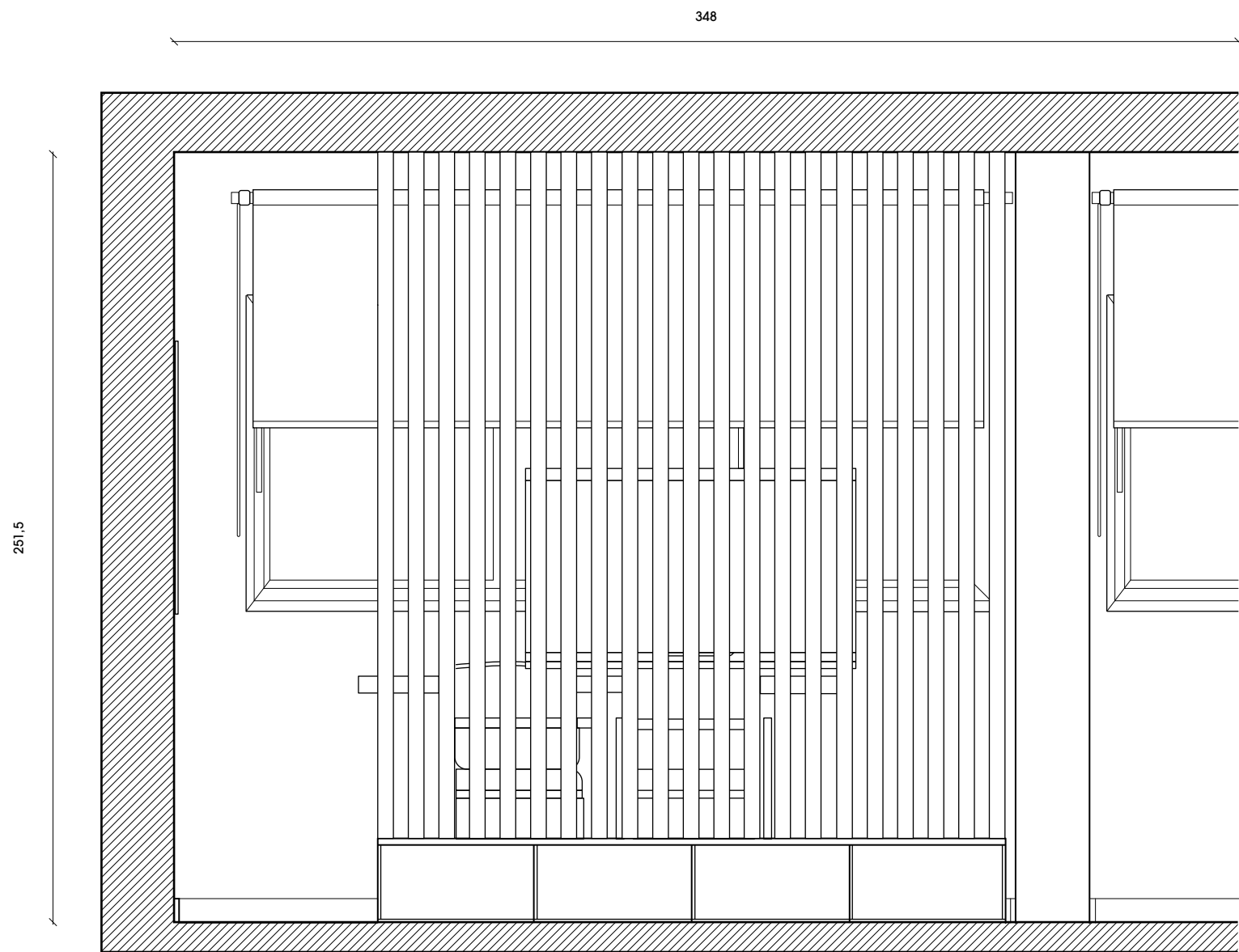
CORTE GH
