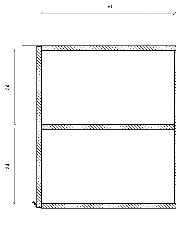
CORTE AB
