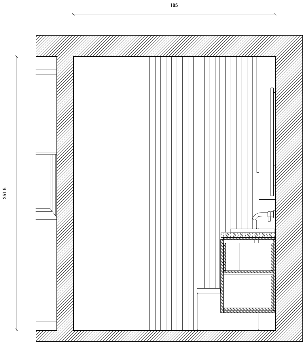
CORTE CD
