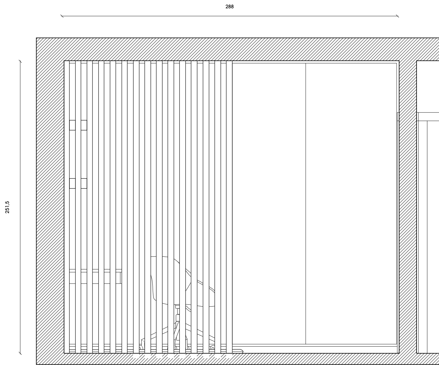
CORTE EF
